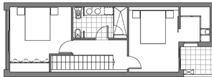
Plantes baixa, primera i segona
